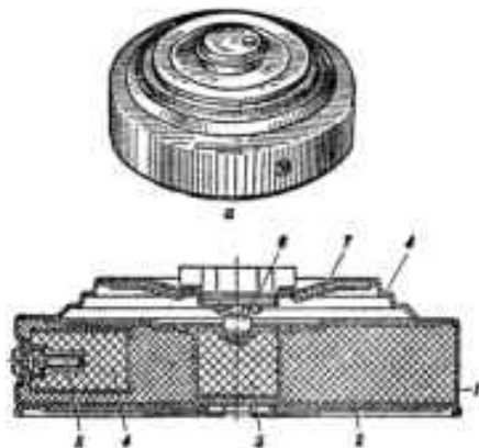
Минаи зиддитанкии ТМ-57
