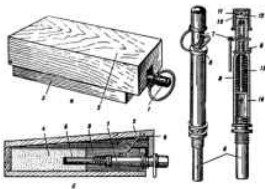
Минаи зиддипиёдагарди ПМД-6М
